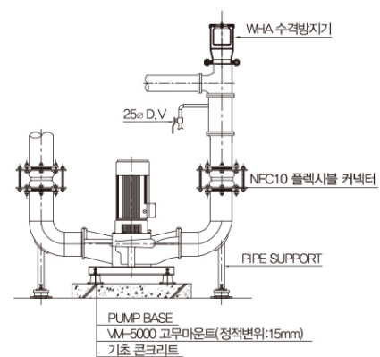
인라인 펌프 방진 상세도
