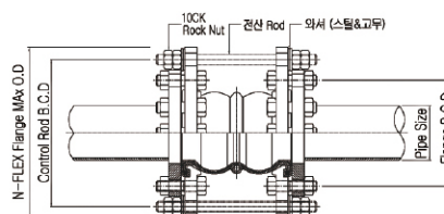
CONTROL ROD 설치상세도
