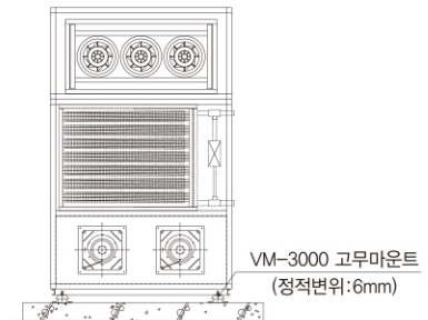
제트 공기조화기 방진 상세도
