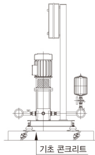
기초 콘크리트
