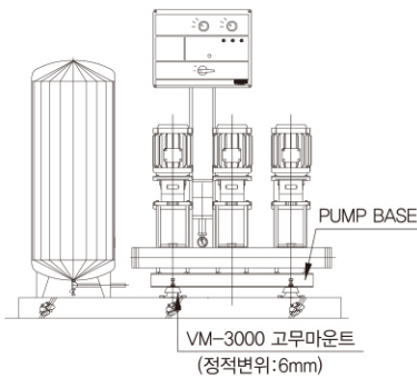
부스타펌프 방진 상세도
