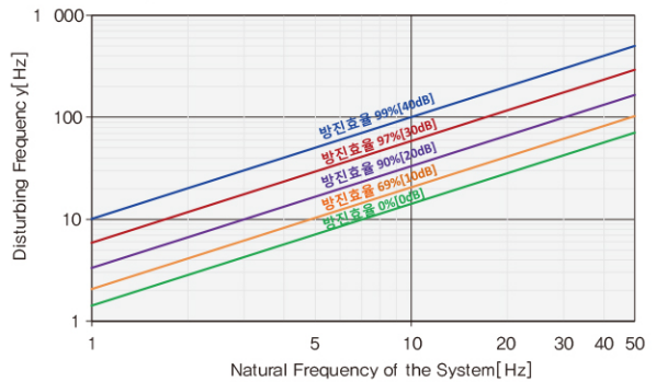
방진효율계산서
