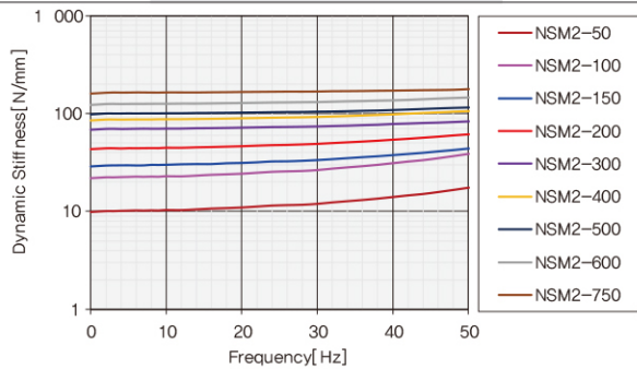
동강성 Graph
