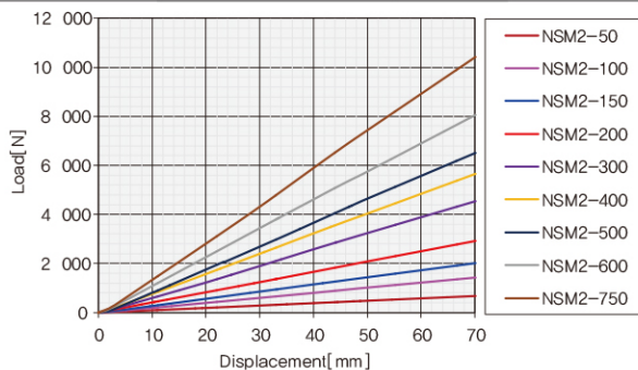
하중-변위 Graph
