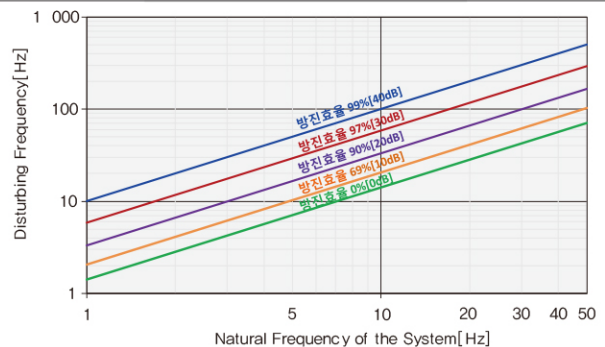
방진효율계산서
