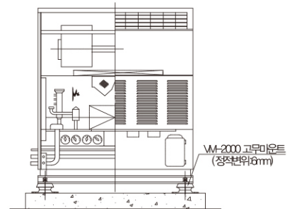
항온 항습기 방진 상세도
