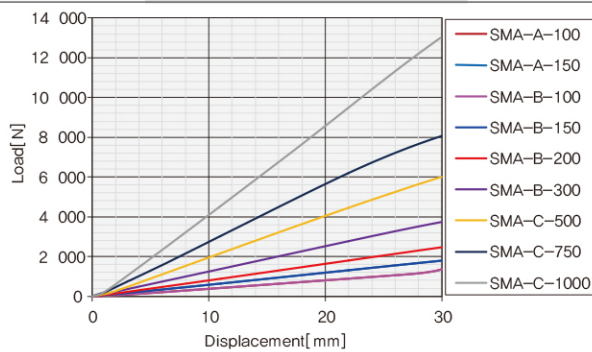
하중 변위 Graph
