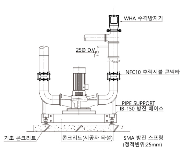
인라인 펌프 방진 상세도
