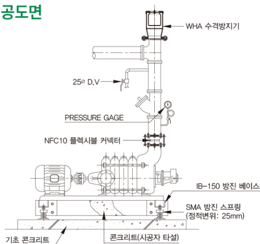
다단볼류트 펌프 방진 상세도
