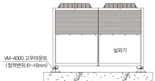
E.H.P 실외기 방진 상세도
