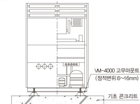
팩케이지 에어컨 방진 상세도
