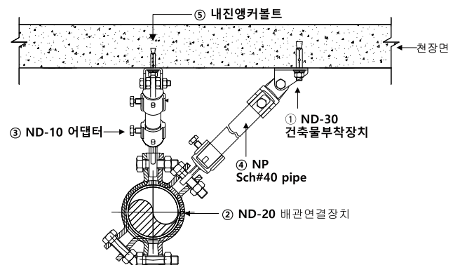
〈수평배관〉
