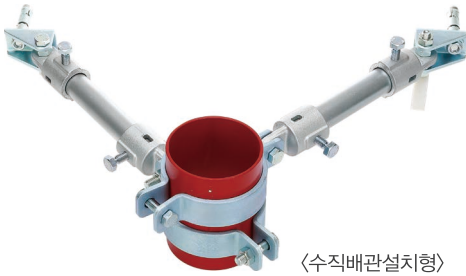
〈수직배관설치형〉
