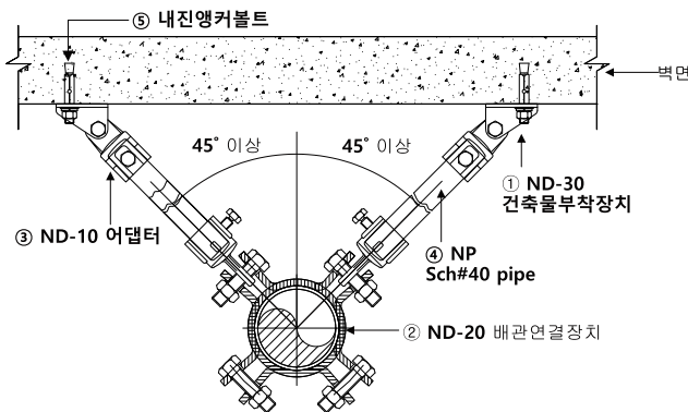
〈수직배관〉
