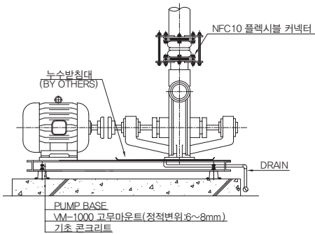
웨스코 펌프 방진 상세도
