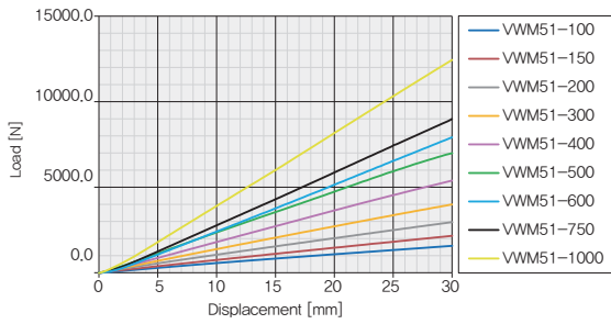
하중-변위 Graph
