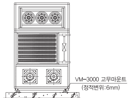
제트 공기조화기 방진 상세도
