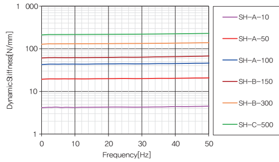
동강성 Graph
