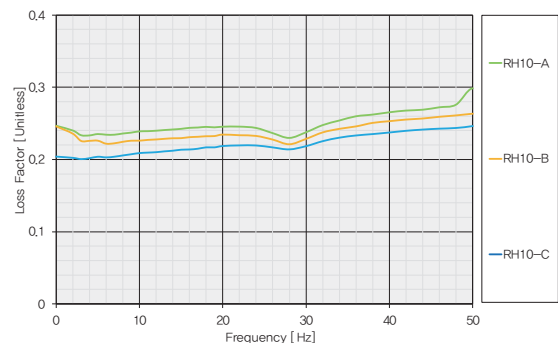
방진효율계산서
