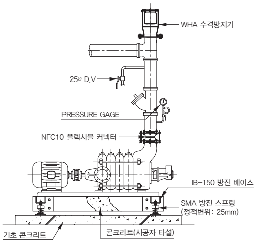
다단볼류트 펌프 방진 상세도
