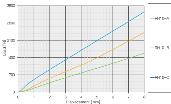
하중-변위 Graph
