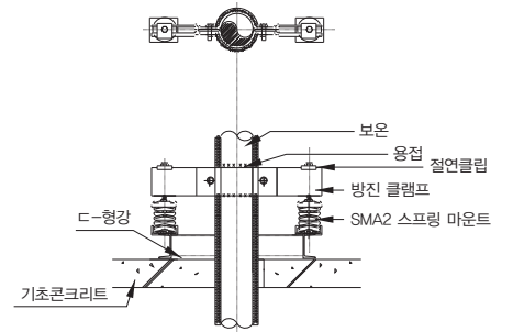
방진 스프링 설치상세도
