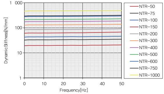
동강성 Graph
