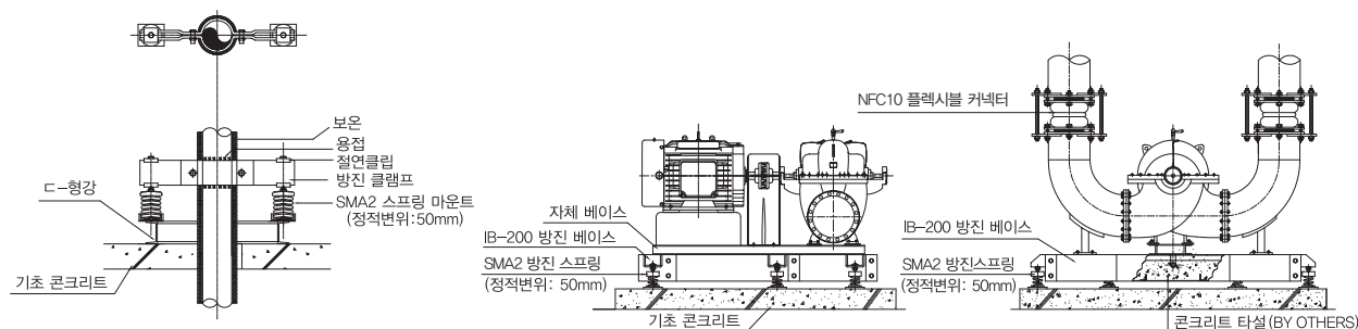
입상 방진 스프링 설치상세도
