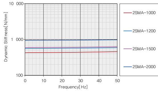
동강성 Graph
