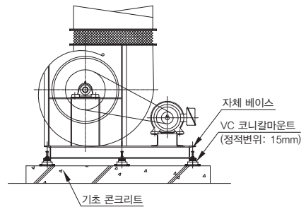
송풍기 방진 상세도
