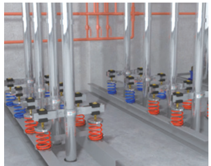
방진 스프링 설치 완료
