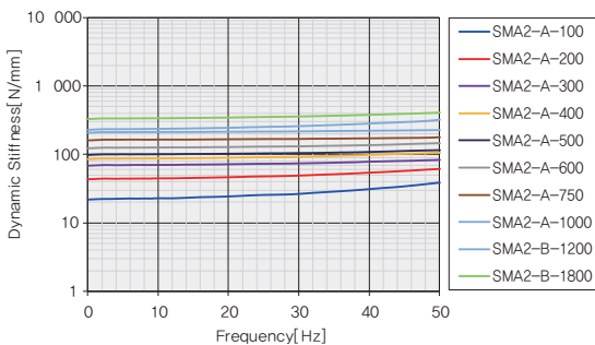
동강성 Graph
