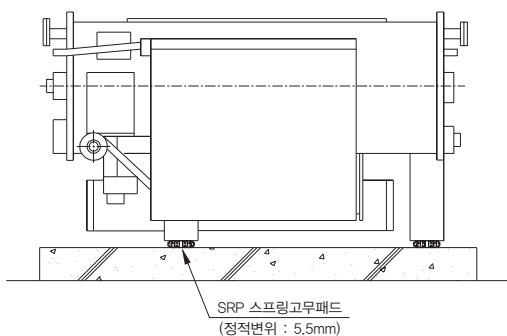
흡수식 냉동기 방진 상세도
