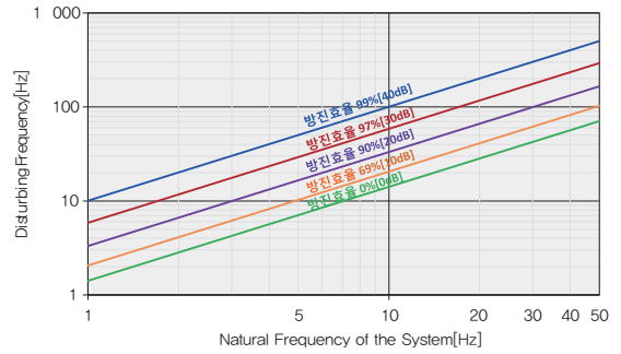
방진효율계산서
