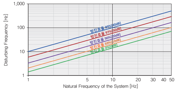
방진효율계산서
