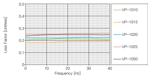
손실계수 Graph
