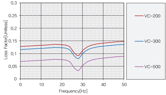
방진효율계산서
