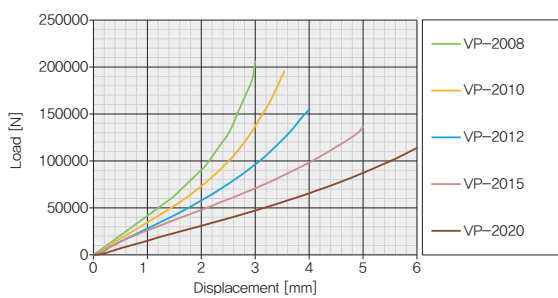
하중-변위 Graph
