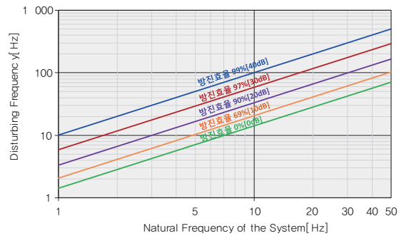
방진효율계산서
