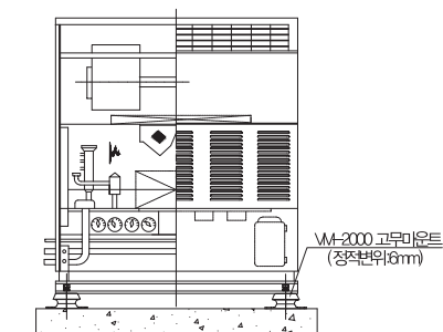
향온 향습기 방진 상세도
