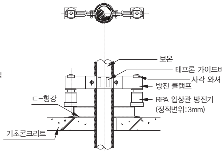
방진 가이드 설치상세도
