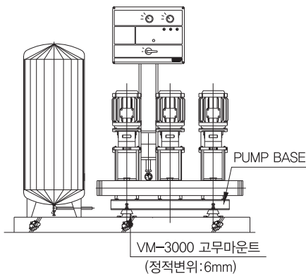
부스타펌프 방진 상세도
