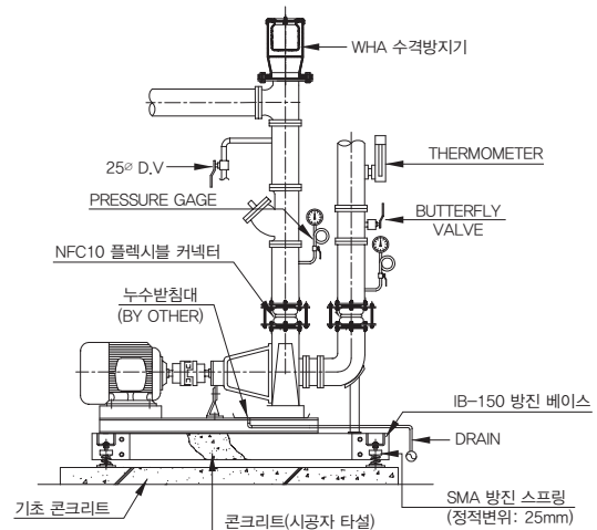
단단볼류트 펌프방진 상세도
