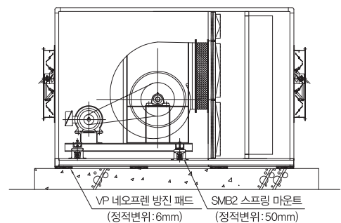
배기탈취 유니트 방진 상세도
