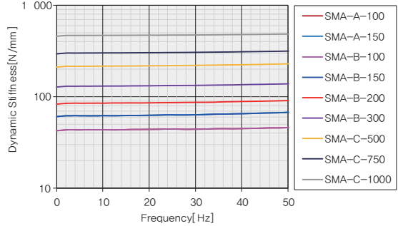
동강성 Graph
