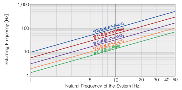
방진효율계산서
