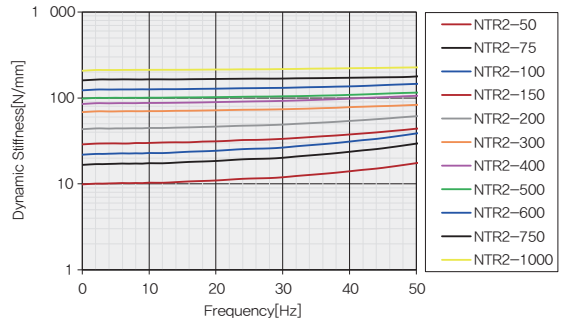
동강성 Graph
