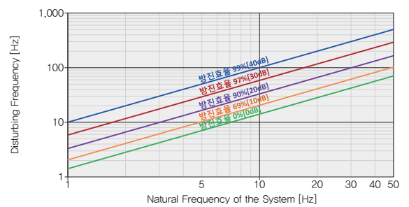
방진효율계산서
