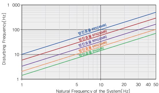
방진효율계산서
